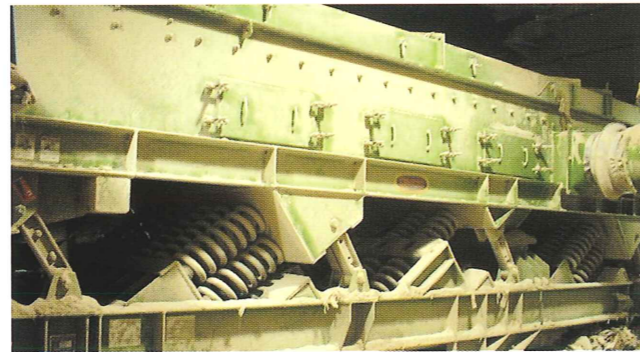
東京都 江東区 T社 建設廃材選別装置
