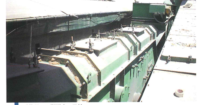
千葉県 四街道市 T社 建設廃材選別装置
