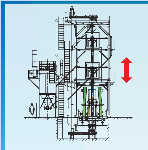
投射部内部
