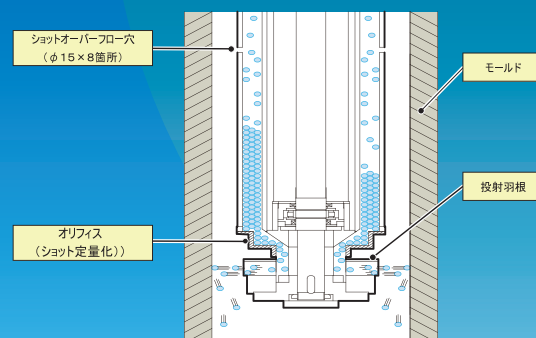
投射部内部
